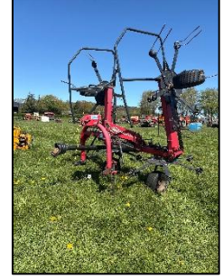
Vicon Fanex X-524 4 x Rota Tedder - £2,800
